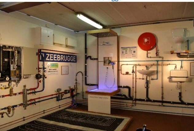
6 Installatie VTI-Zeebrugge
