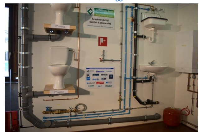
8 Installatie VTI-Zeebrugge
